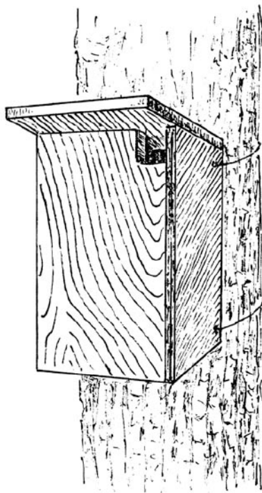
Рис. 3. Синичник с угловым квадратным летком.
