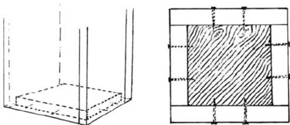
Рис. 5. Способ крепления дна дуплянки. Дно должно находиться внутри стенок гнездовья.
