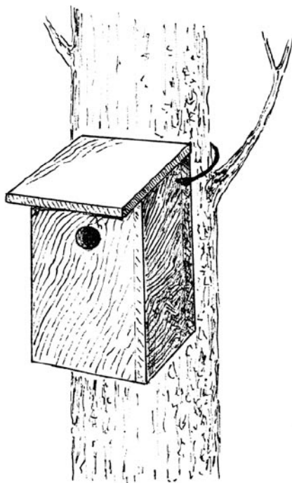
Рис. 7. Способ закрепления дуплянки на дереве.
