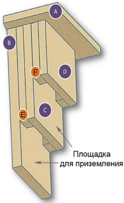
Домик для летучих мышей типа Kent-box
